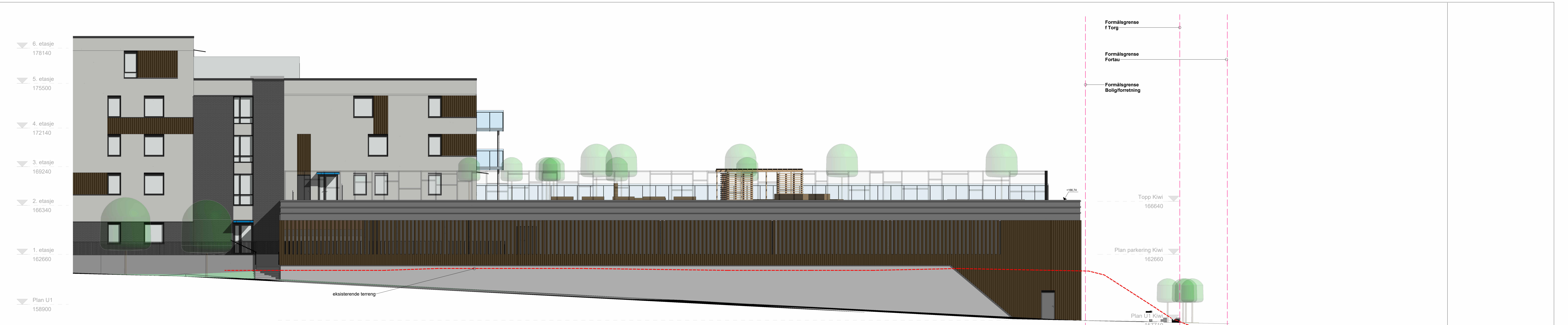
Rammesøknad KIWI fasade nord-øst 1 : 100
